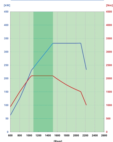
CURSOR 10 - 450HP E4/E5
